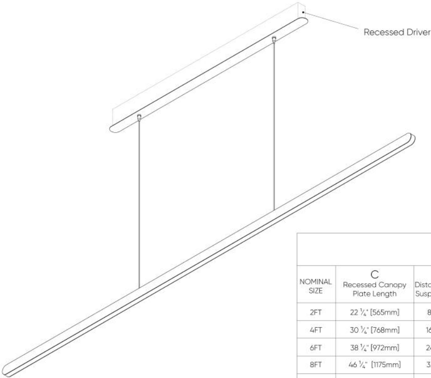
LUMINAIRE DIMENSIONS
